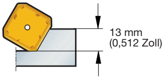
Maximale Schnitttiefe für Plattengröße 19 mm
