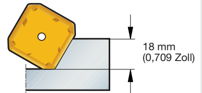
Maximale Schnitttiefe für Plattengröße 28 mm
